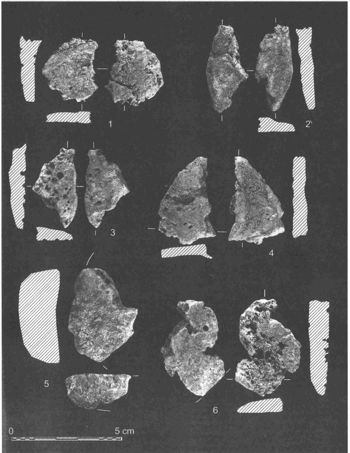
Рис. 2.17. Слитки черновой и рафинированной меди
