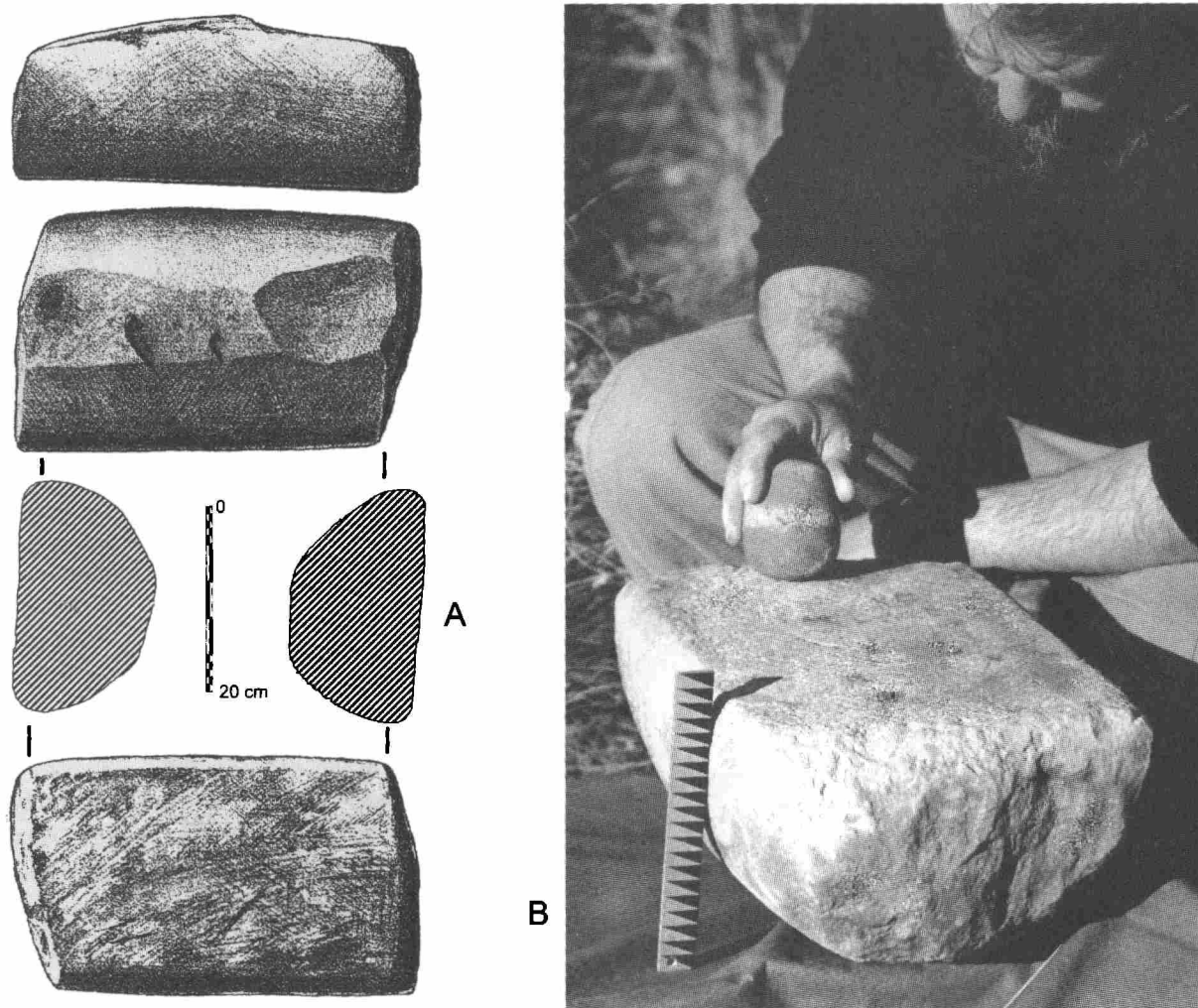
Рис. 6.13. Наковальня из монолита кристаллической породы: A – рисунок изделия, B – его фото; кв.4627, близ обваловки плавильного двора комплекса №1, субфаза B-1 ; вес 36, 68 кг [см. также: Каргалы, том 2, с. 79–80, рис. 3.11–3.13]
