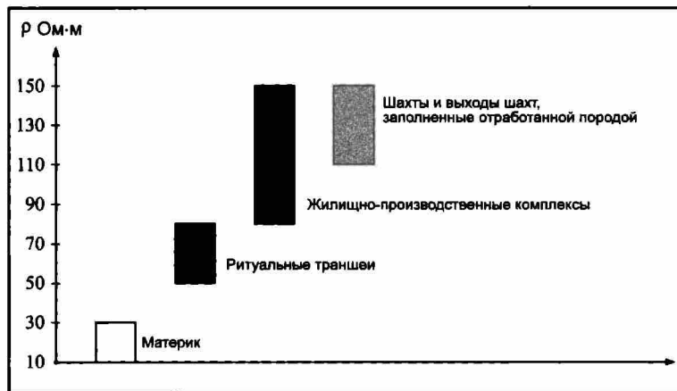
Рис. Пр.3.4. Поселение Горный. «Шкала сопротивлений» для функциональной интерпретации археологических объектов по геофизическим данным
