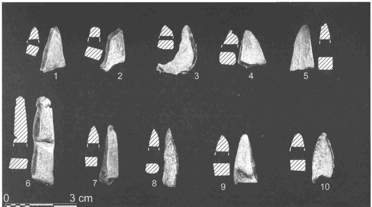
Рис. 2.4. Горнопроходческие орудия: концевые фрагменты кайл-кирок
