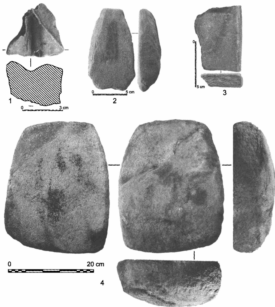
Рис. 5.12. Литейные формы: матрица (наконечник копья) и крышки; песчаник 1 – кв. 4827, субфаза B-3 ; 2 – кв. 3939, комплекс №3, жилище №49, субфаза B-1 ; 3 – кв. 4826, субфаза B-2 ; 4 – кв. 5531, комплекс №2, субфаза B-1
