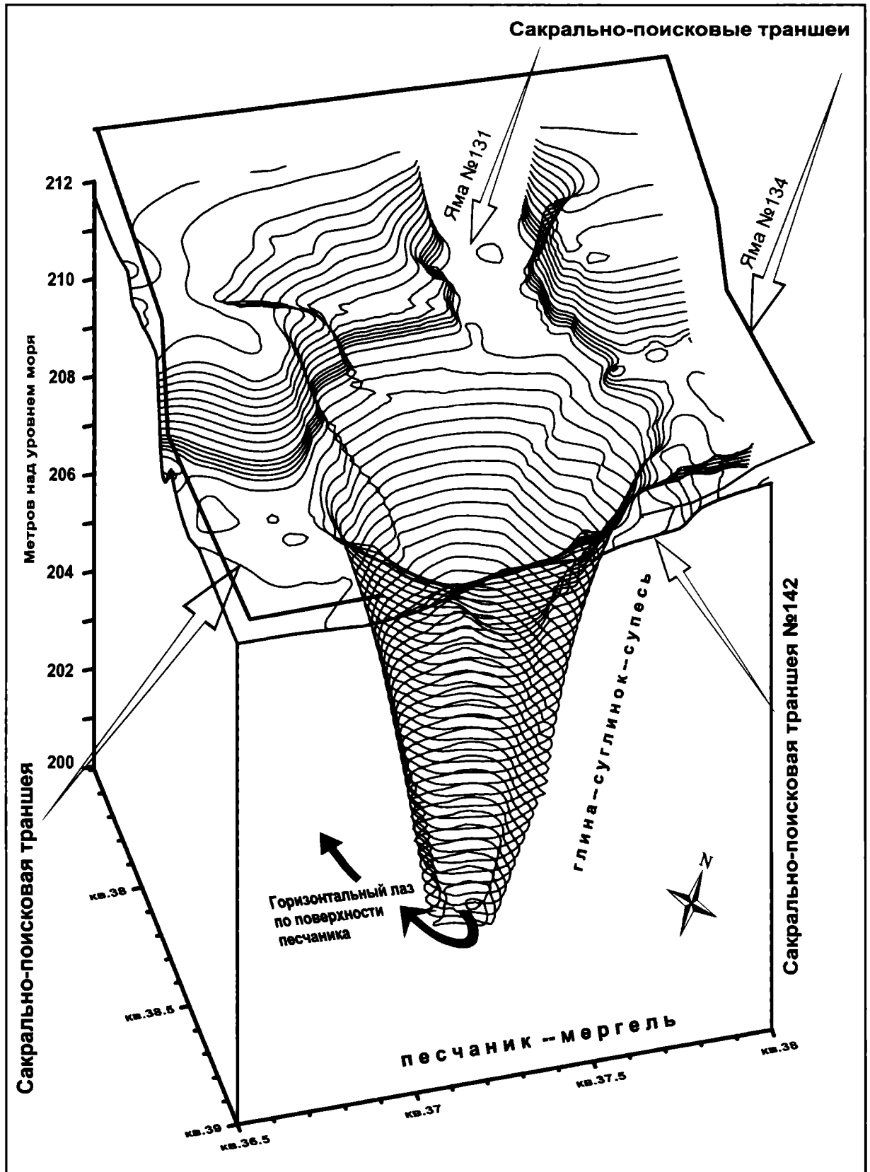
Рис. 9.3. Компьютерная графическая реконструкция конусовидного ствола шахты комплекса №3
