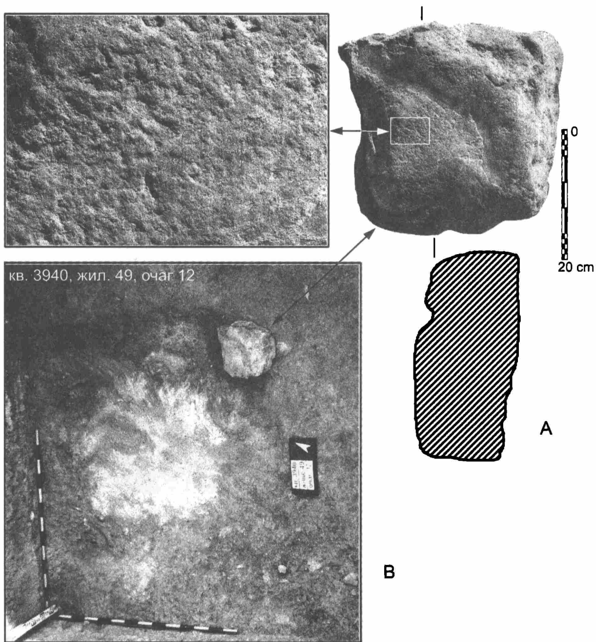
Рис. 6.14. Наковальня на крупном валуне (А), жилище №49, очаг №12, субфаза В-1 (вес 33,4 кг); вверху слева – макрофото участка со следами кузнечных операций поверхности в виде мелких выбоин; внизу слева (В) – положение наковальни in situ близ золистого пятна очага
