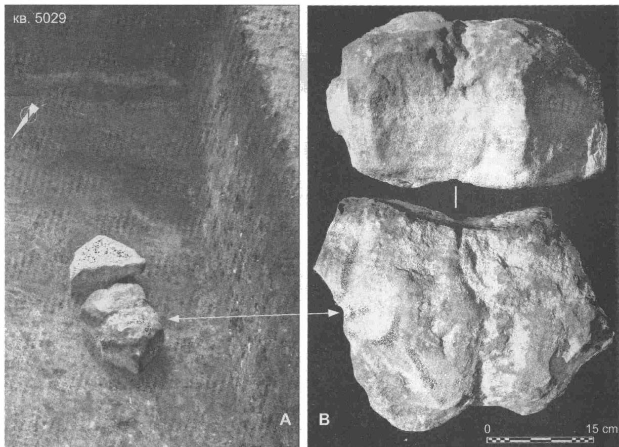
Рис. 6.17. Массивный песчанниковый противовес «колодезного» типа. A – положение обеих сохранившихся его частей в культурном слое селища; B – центральная часть противовеса, где отчетливо виден желоб для обвязки его канатом или кожаным ремнем (лентой)
