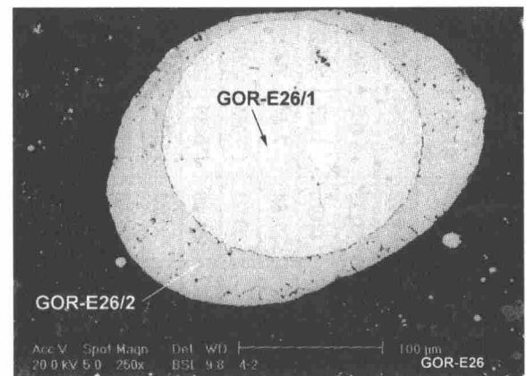
Рис. 4.3. Микроструктуры образцов шлака (1–6). Магнетитовые кристаллы в шлаке (4)
