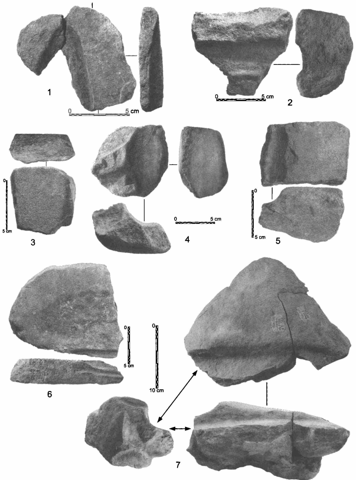
Рис. 5.6. Литейные формы: кайла-кирки; песчаник
