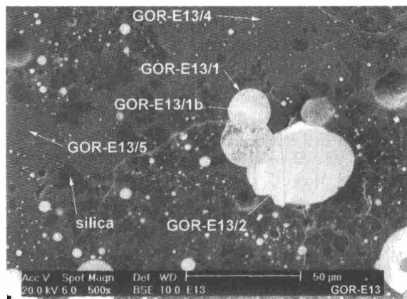
Рис. 4.3. Микроструктуры образцов шлака (1–6). Магнетитовые кристаллы в шлаке (4)
