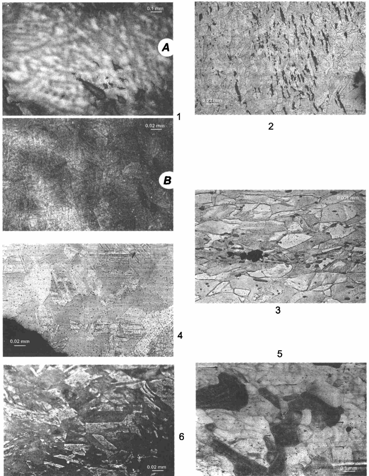
Рис. 4.6. Микроструктуры образцов различных медных изделий:
