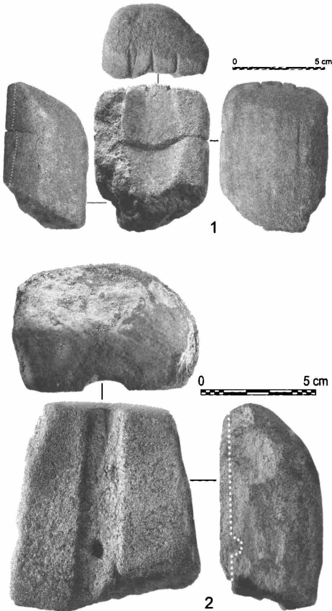
Рис. 5.7. Литейные формы: нож (1) и нож-кинжал (2); песчаник 1 – кв. 4929, субфаза В-3; 2 – кв. 3839, субфаза В-3
