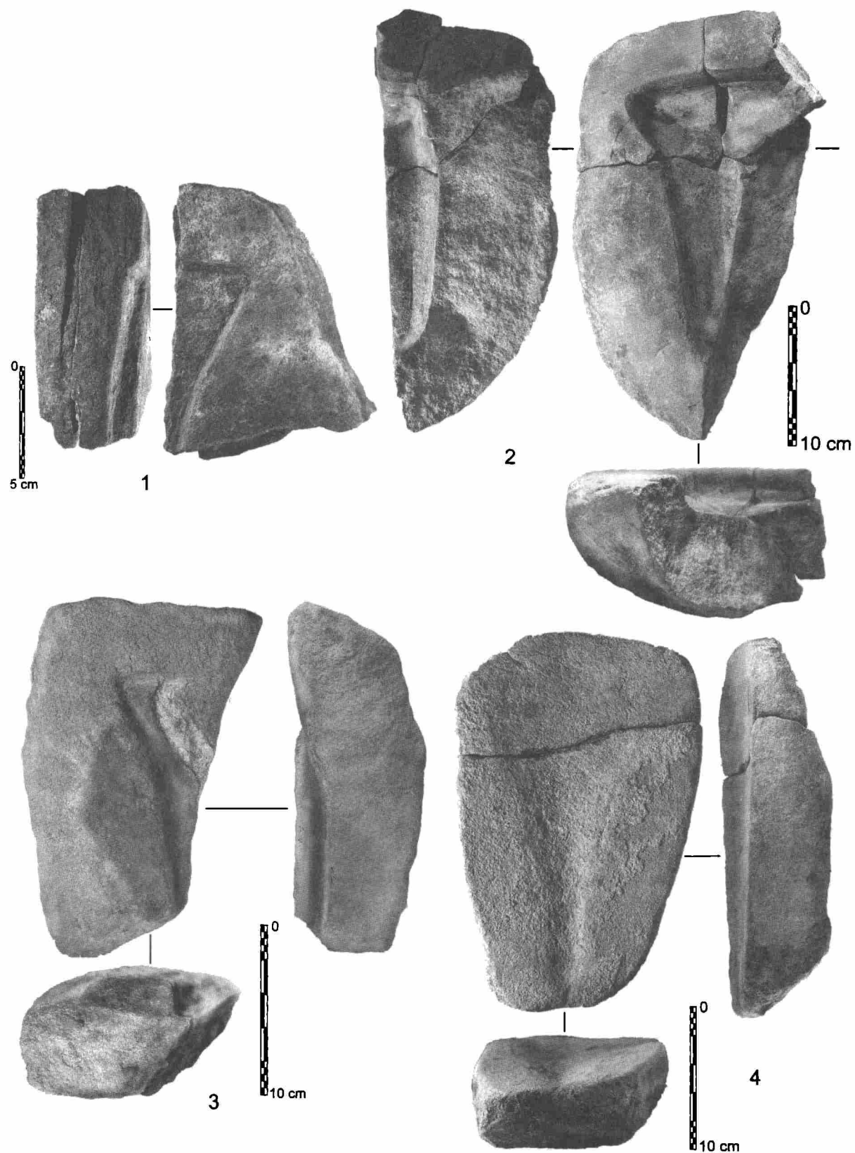
Рис. 5.2. Литейные формы: кирки-пешни; песчаник
