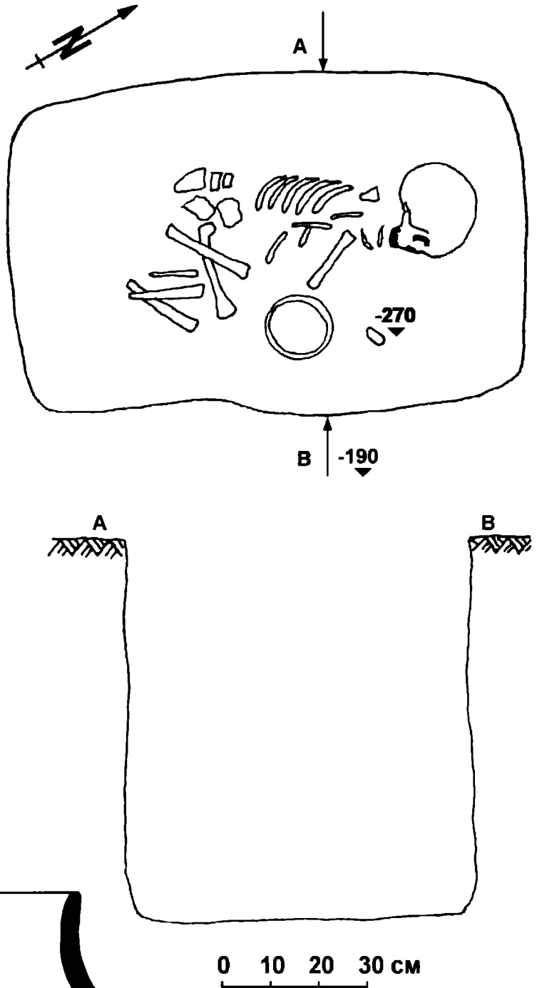
Рис. 3.15. Комиссарово, курган №1: погребение №7
