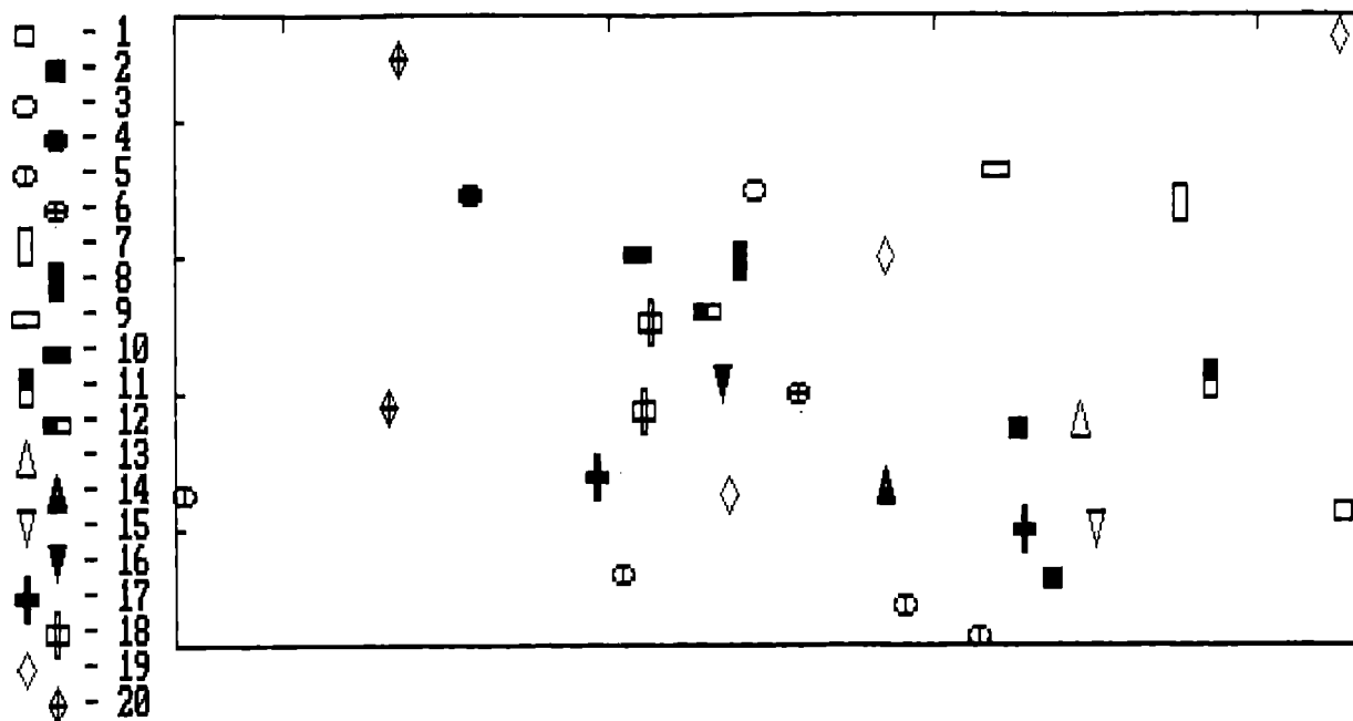
Рис. 8.2. Итоги канонического анализа межгрупповой изменчивости признаков посткраниального скелета у мужчин эпох энеолита и бронзы в плоскости первой и второй канонической переменных.
