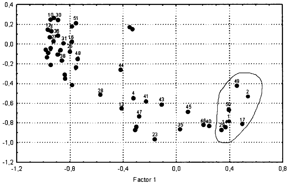
Рис. 7.6. Расположение исследованных групп в пространстве I и II главных компонент по 5 признакам. Обозначение групп согласно нумерации в табл. 7.3
