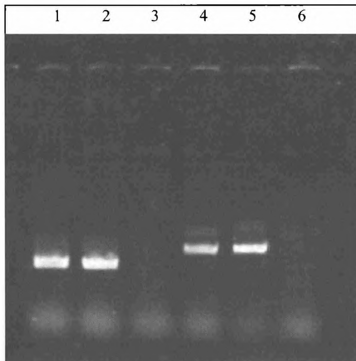
Рис. 12.1. Молекулярно-генетическое определение пола у индивида из погребения 4 Першинского кургана (образец №20). Дорожки 1–3 – амплификация фрагмента митохондриальной ДНК (L15989-H16190, длина 239 п.н.). 1 – образец №20, 2 – положительный контроль (современная ДНК), 3 – отрицательный контроль выделения. Дорожки 4–6 – амплификация Y-специфичного повтора DYZ1 (длина ампликона 305 п.н.). 4 – образец №20, 5 – положительный контроль (современная ДНК), 6 – отрицательный контроль выделения. Видны отчетливые специфические сигналы в обеих системах. Отсутствие сигнала в отрицательных контролях свидетельствует об аутентичности полученных данных.
