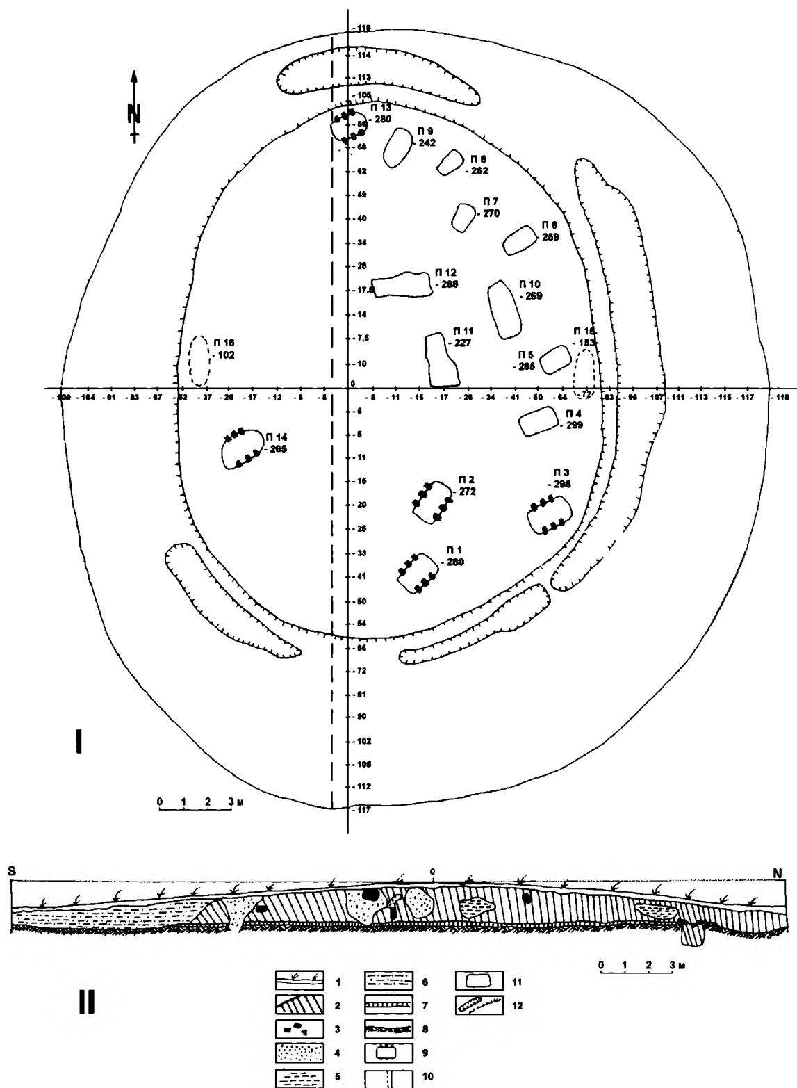
Рис. 3.2. Комиссарово, курган №1: общий план (I) и профиль бровки (II).
