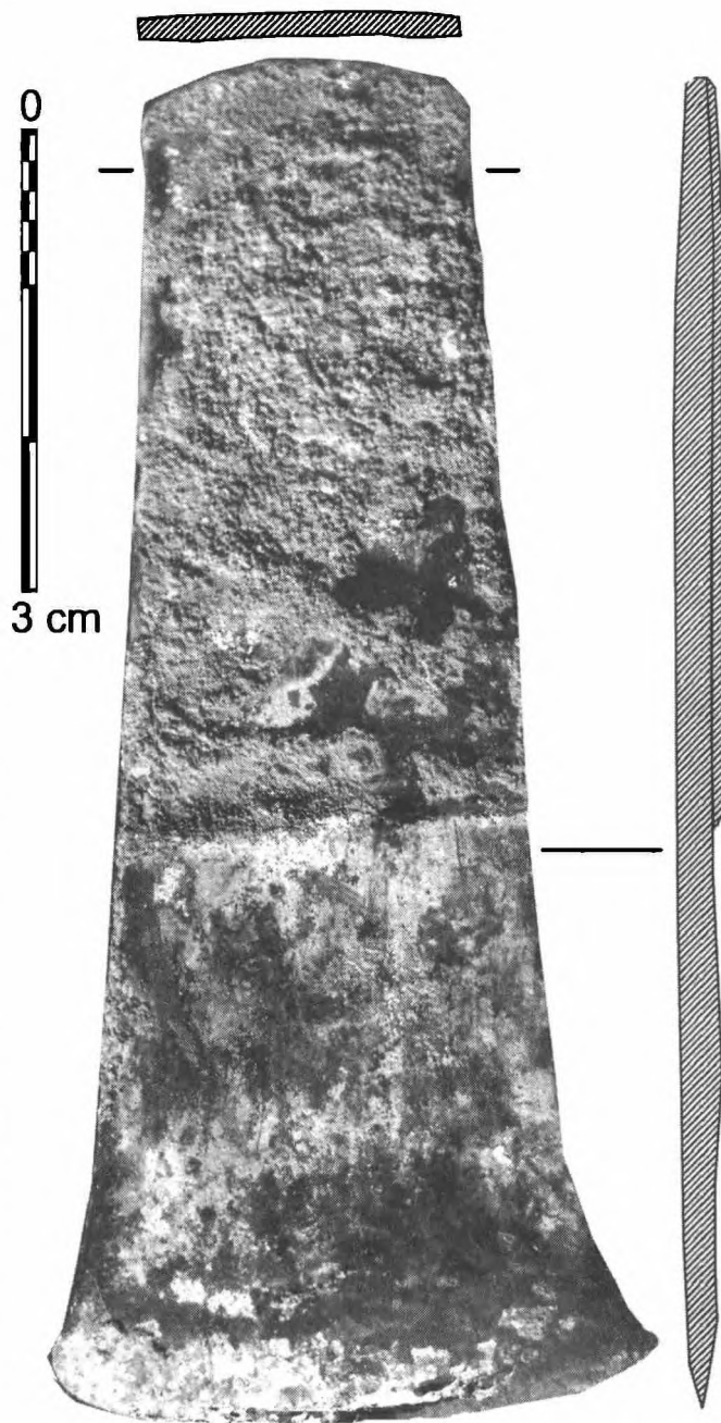
Рис. 1.34. Першин, курган №1: медное тесло из курганной насыпи (вне погребений)
