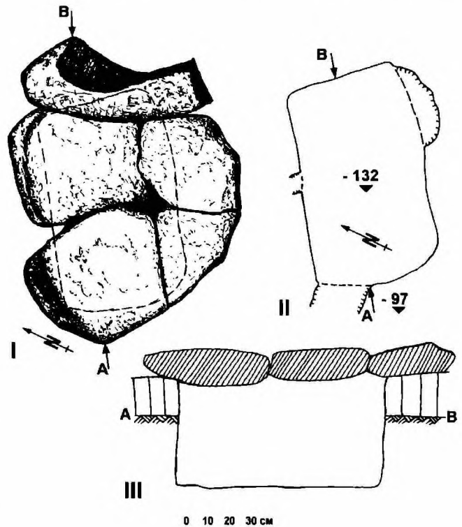
Рис. 2.5. Першин, курган №3: погребение №2
