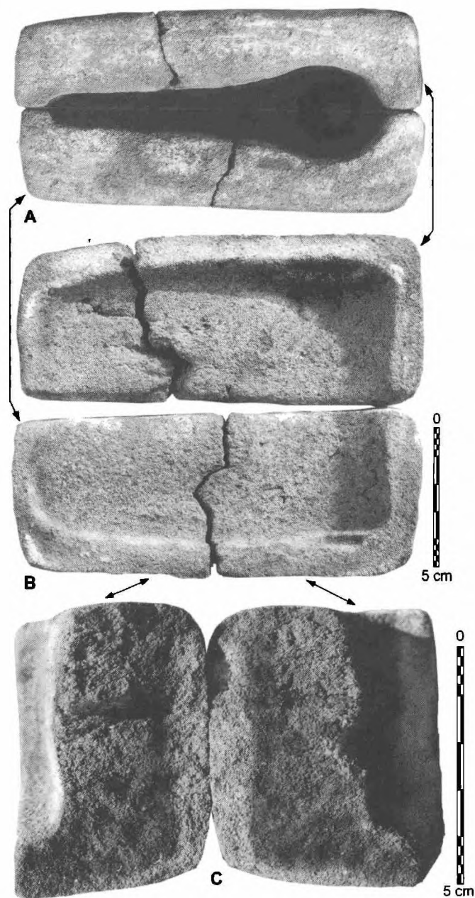
Рис. 1.13. Першин, курган №1: глинисто-песчановая литейная форма для втульчатого топора из погребения №4; две намеренно расколотые створки (А); сложенные вместе створки с литником, но без сердечника (В); следы сильного внутреннего прокала на изломе одной из створок (С)
