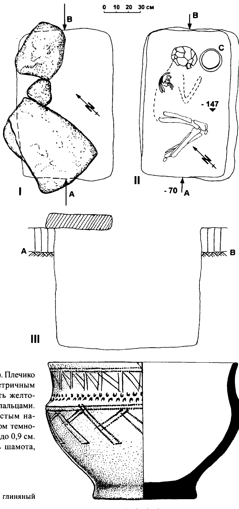
Рис. 2.12. Першин, курган №3: погребение №6
