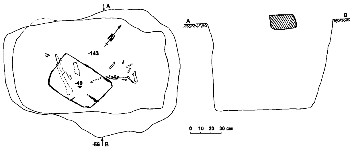
Рис. 3.38. Комиссарово, курган №2: погребение №3
