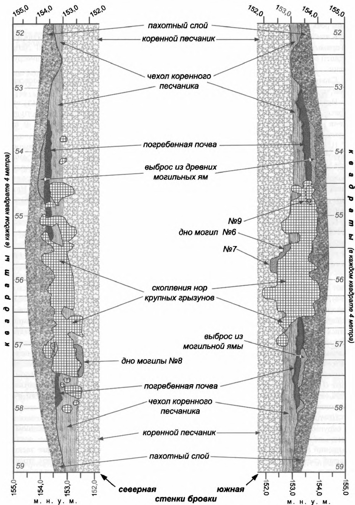
Рис. 1.8. Першин: профильные – северная и южная – стенки (разрезы) центральной бровки кургана №1
