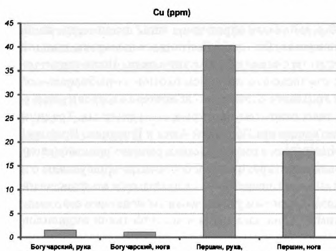
Рис. 11.1. Концентрации меди в костной ткани индивидов из погребений Богучарского и Першинского могильников
