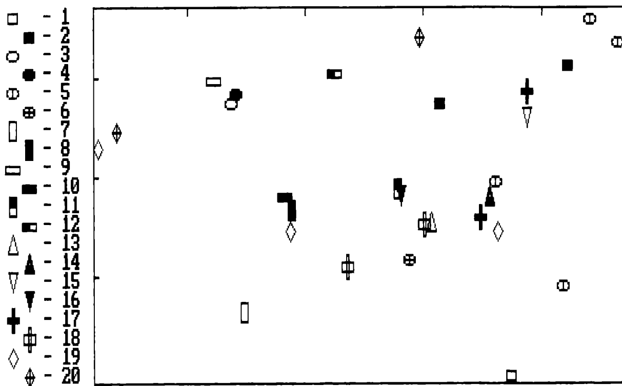
Рис. 8.4. Итоги канонического анализа межгрупповой изменчивости признаков посткраниального скелета у мужчин эпох энеолита и бронзы в плоскости второй и третьей канонической переменных.
