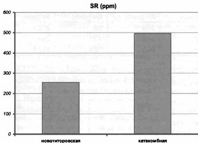
Рис. 11.2. Концентрации стронция в костной ткани индивидов из погребений новотиторовской и катакомбной культур
