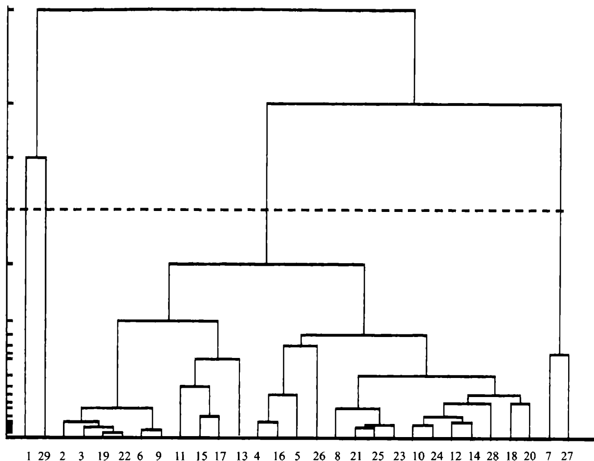
Рис. 8.5. Результаты кластерного анализа с учетом таксономической ценности признаков.
