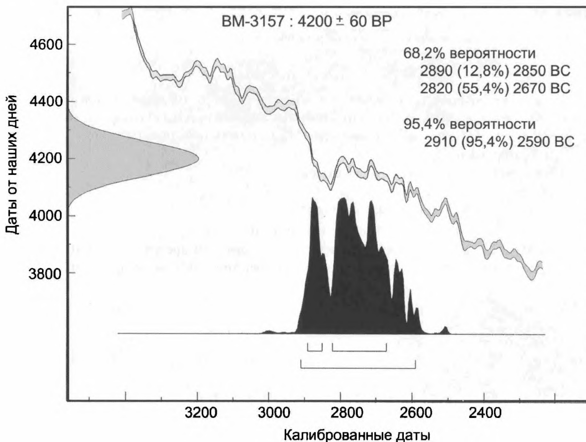
Рис. Пр.2.1. Распределение вероятностей калиброванных значений возраста дерева из перекрытия могилы №4 Першинского кургана №1
