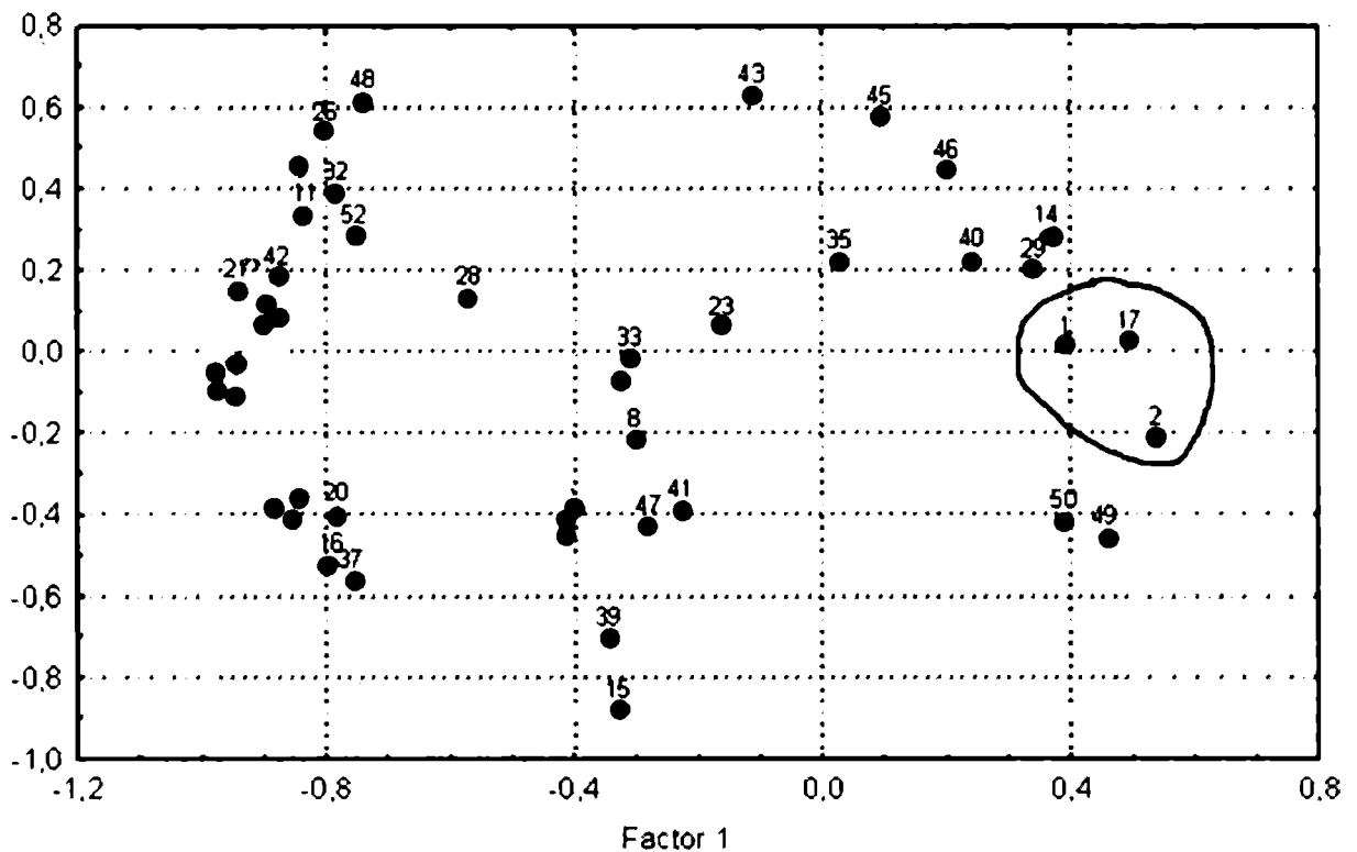
Рис. 7.7. Расположение исследованных групп в пространстве I и III главных компонент по 5 признакам. Обозначение групп согласно нумерации в табл. 7.3
