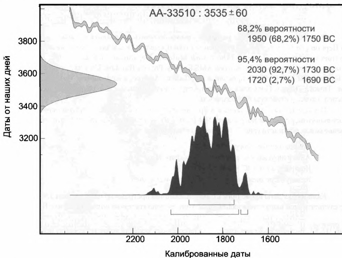
Рис. Пр.2.2. Распределение вероятностей калиброванных значений возраста кости козленка из могилы №2 Першинского кургана №1
