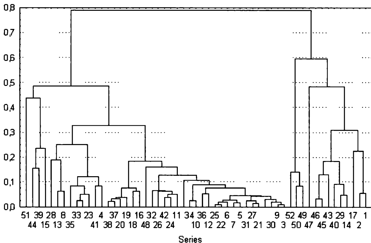
Рис. 7.9. Расположение исследованных групп по результатам кластерного анализа (по 11 признакам). Обозначение групп согласно нумерации в табл. 7.3
